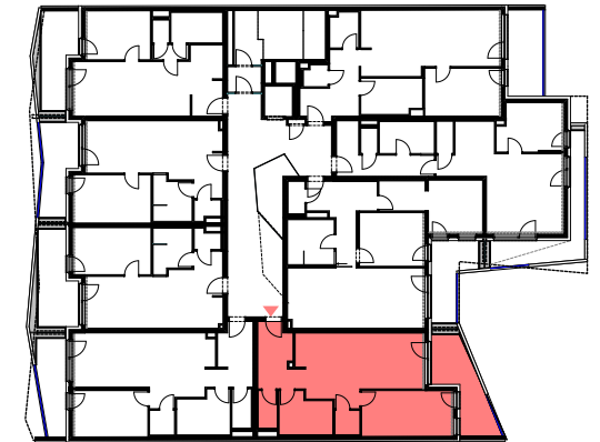
Übersichtsplan OG 4
